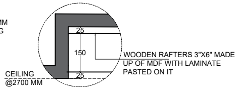
DETAIL Y
